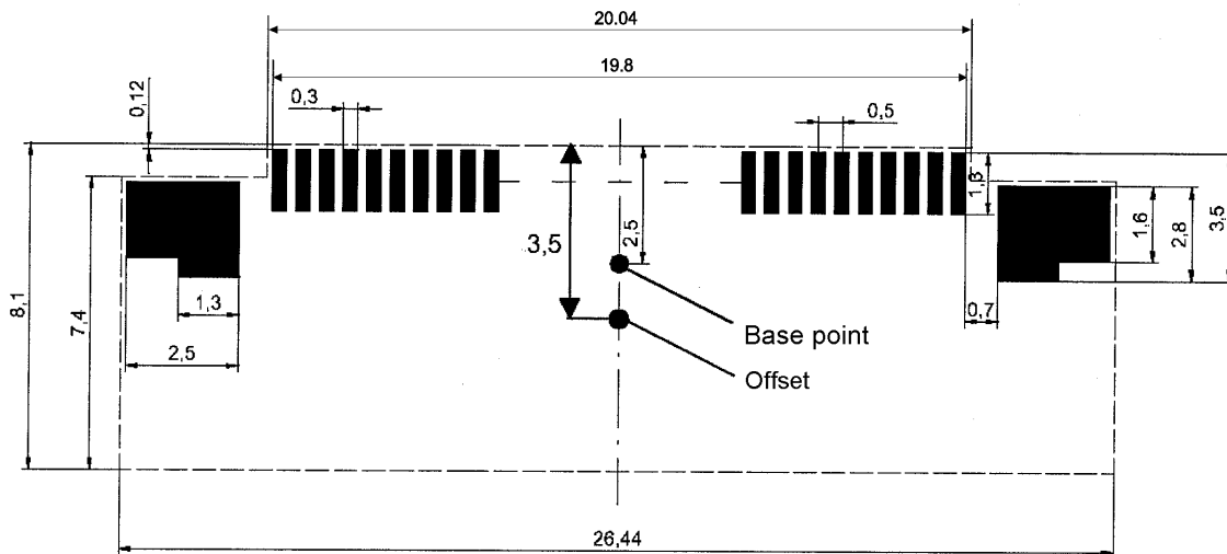
Figure 32: PCB ZIF connector
