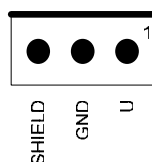
Obrázek 36 – Zapojení vstupů AIn1 až AIn3 (JP9 až JP11)
