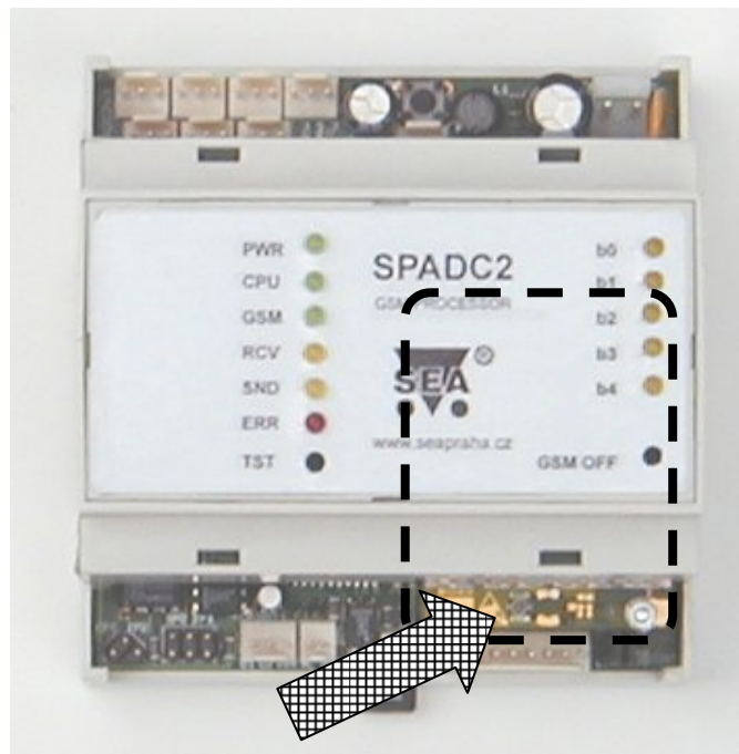
Obrázek 43 – GSM modem a pozice anténního konektoru
