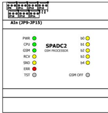
Obrázek 39 – Umístění konektorů JP9 až JP15 (Analogové vstupy)
