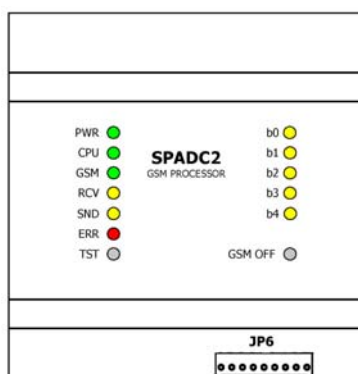
Obrázek 33 – Umístění konektoru JP6 (Digitální vstupy)
