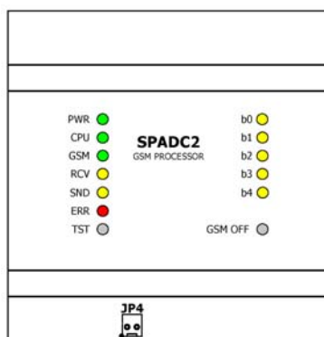
Obrázek 47 – Umístění konektoru JP4 (AC_WATCH)
