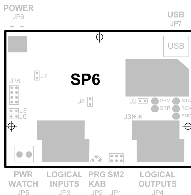
Obrázek 10 – Konektor JP7 pro připojení USB kabelu
