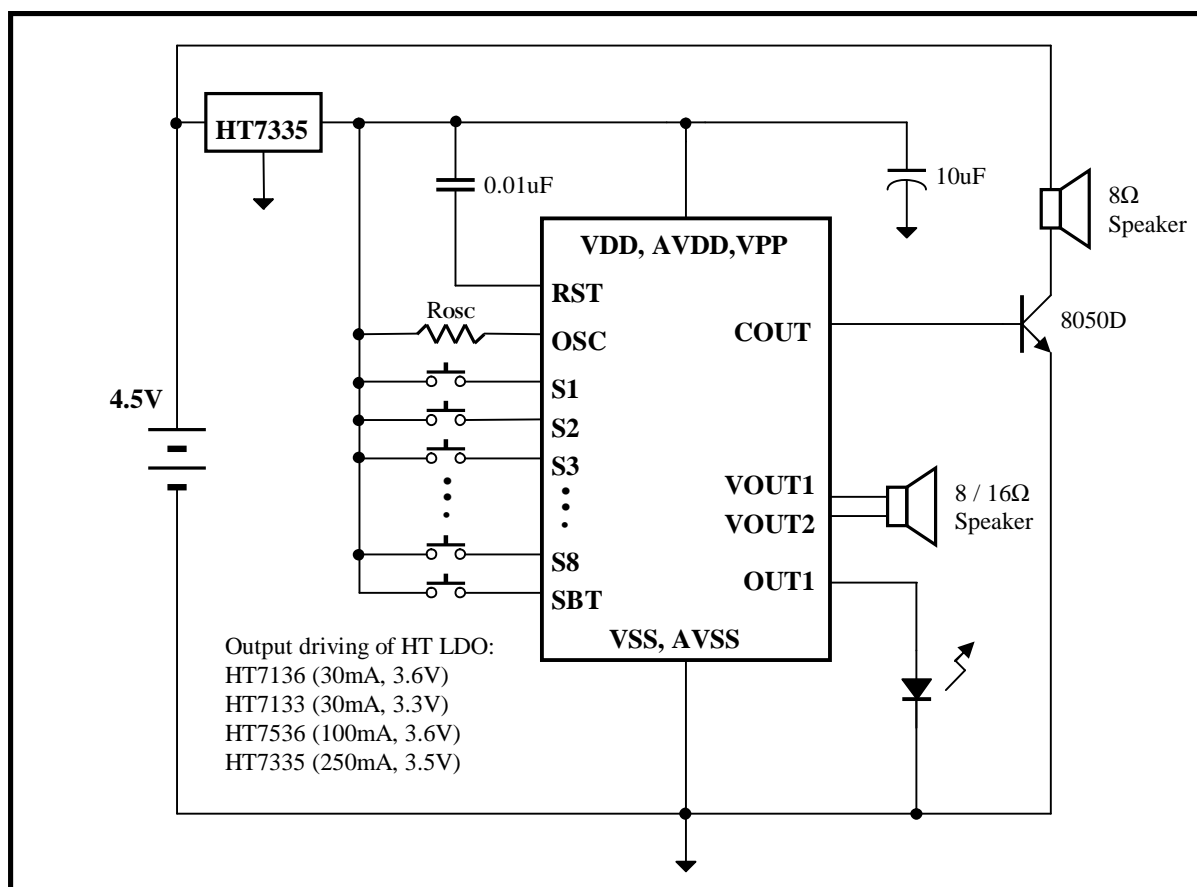
Fig. 23 Using 4.5V Battery
